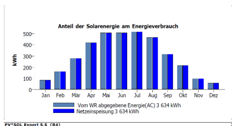
Obrázok 6 Projektovaná mesačná výroba energie vo FVE
